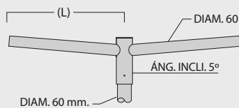
Ref. 821 Cruceta para Luminarias
