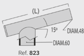
Refs. 823-824 Codos de Conexión
